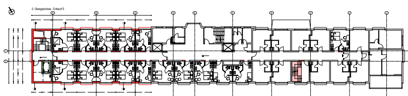
Westflügel, 2. OG
