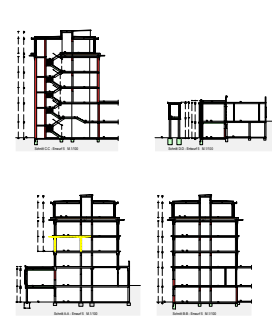
Westflügel, Querschnitt
